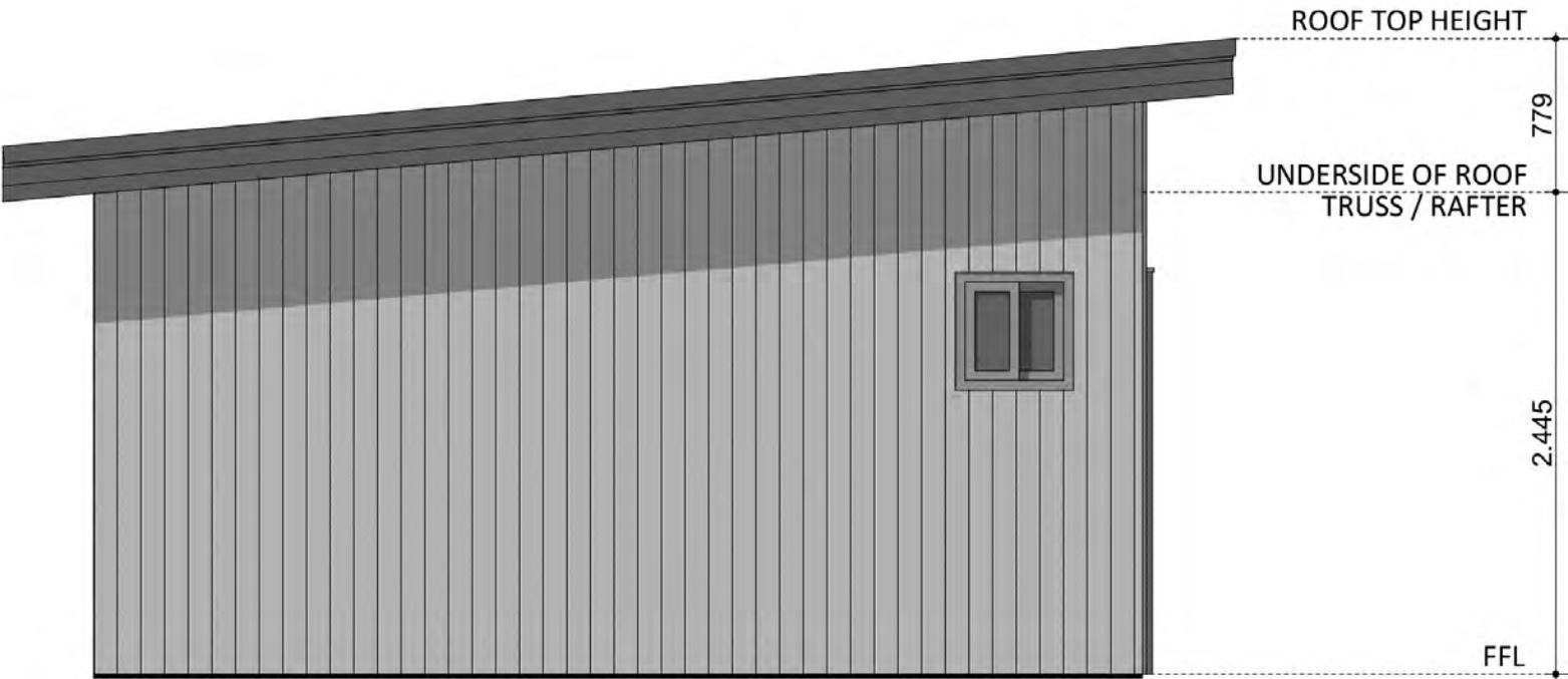
ELEVATION 04
