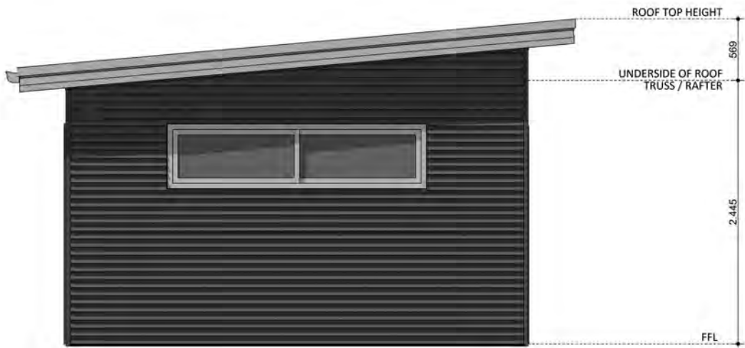
ELEVATION 04
